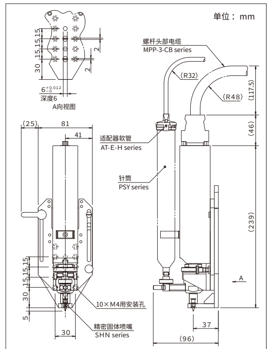
■点胶头部 (MSD-3-SET1时)
