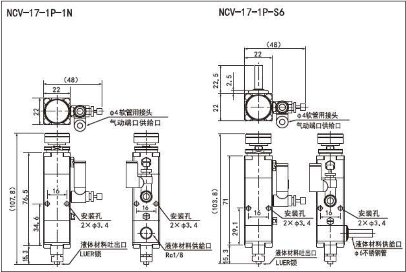
外形尺寸图
