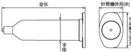
■针筒尺寸图
