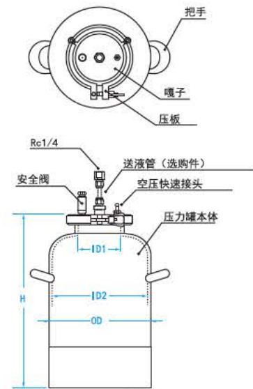
■各部的名称和外形尺寸图
