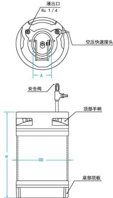
■各部的名称和外形尺寸图
