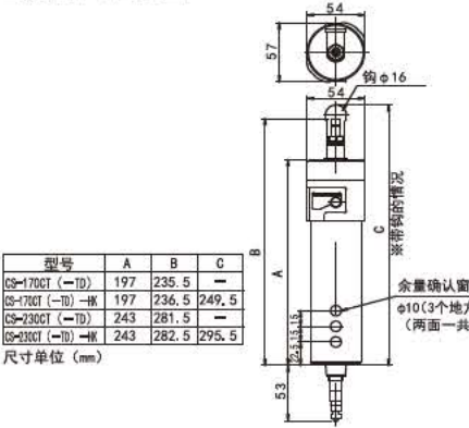
■软管卡筒尺寸图
