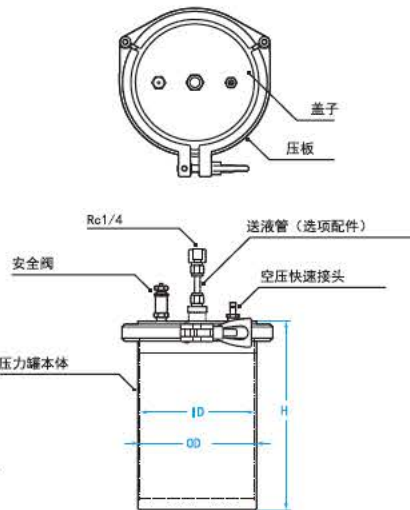
■各部的名称和外形尺寸图
